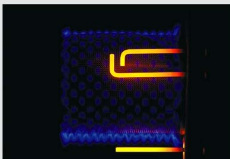
Циліндричний пальник MatriX
