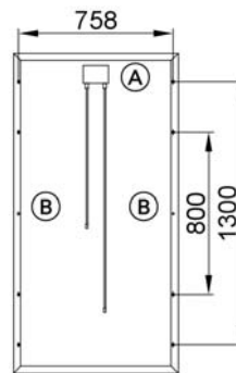
Modulrückseite
