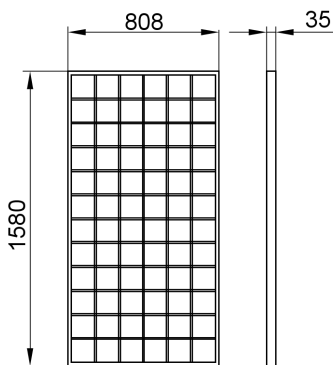
Modulvorderseite
